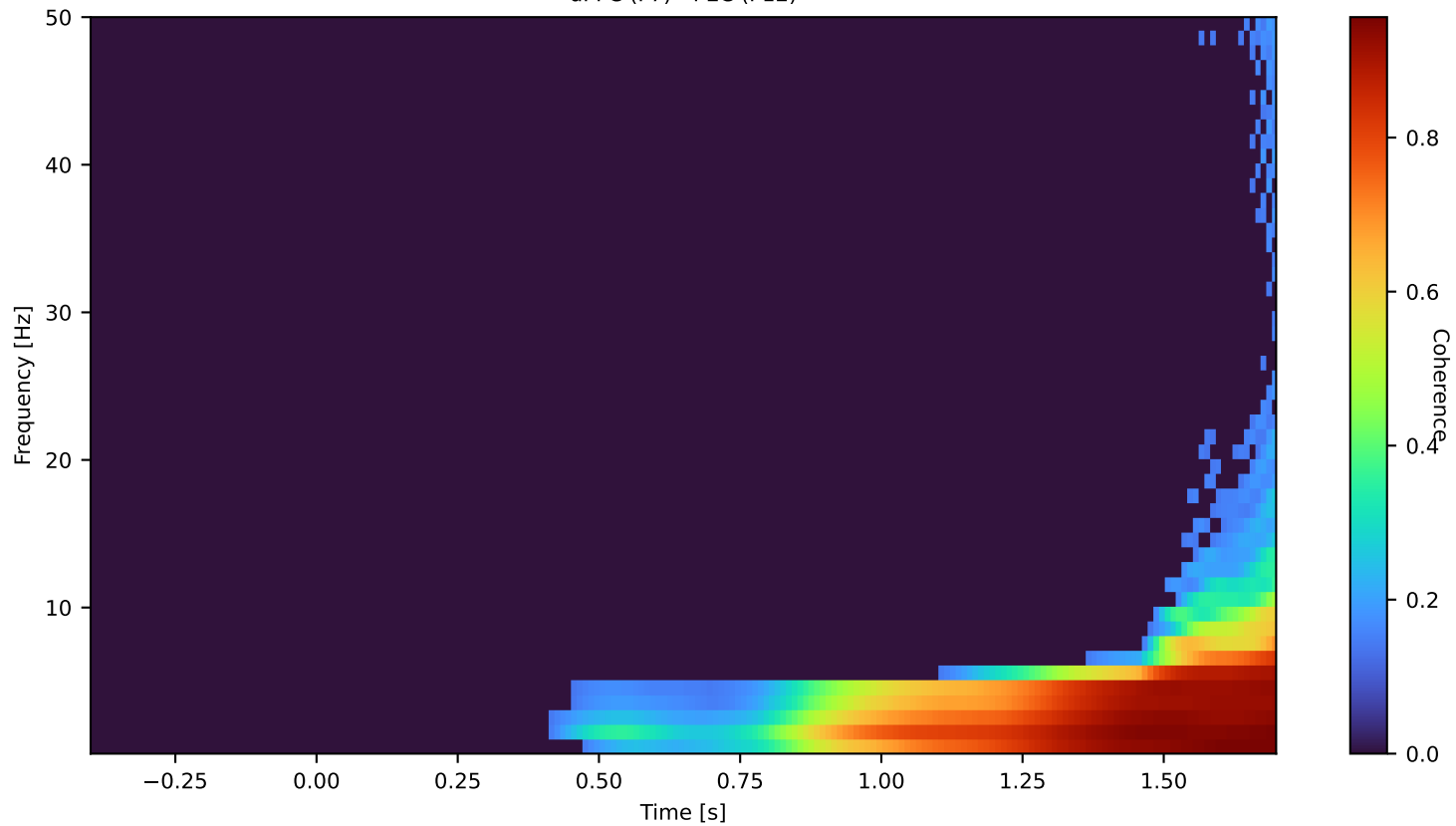
dPFC (F7) - PEC (P12)
